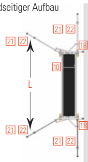
Wandseitiger Aufbau
